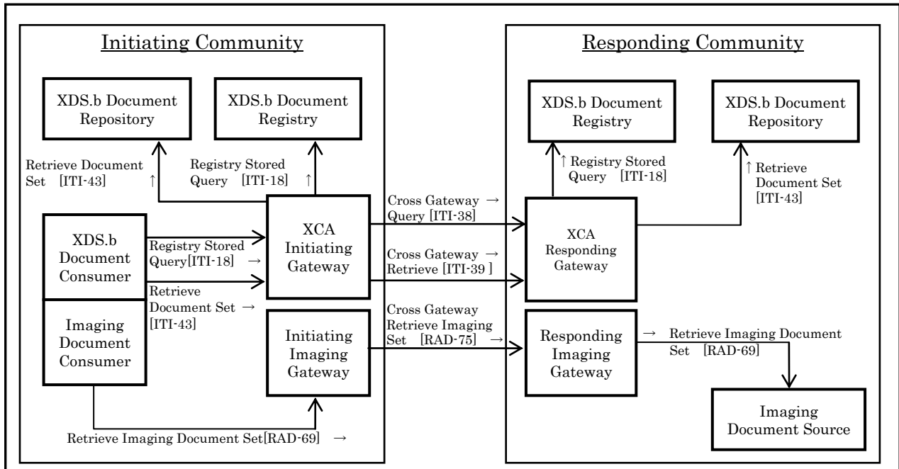
図 17.1 Cross-Community Access for Imaging(XCA-I)のアクタおよびトランザクション
