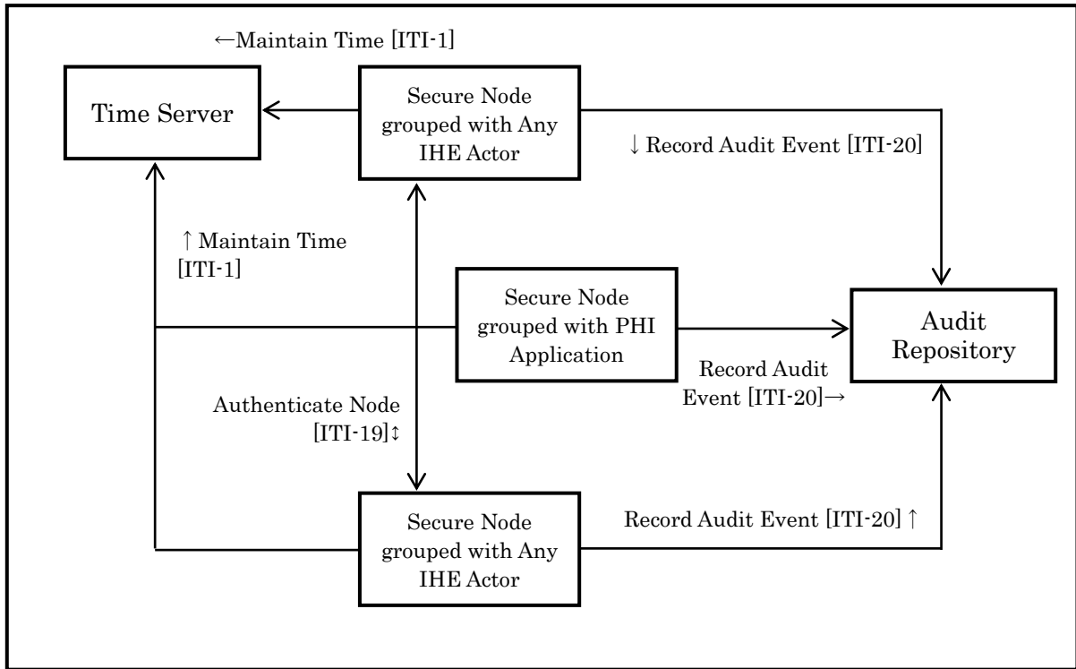
図 16.1 Audit Trail and Node Authentication (ATNA)のアクタおよびトランザクション
