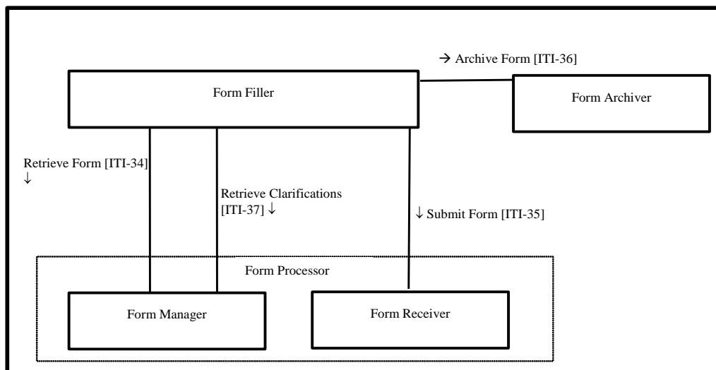
168 169 図 6.1-1: RFD のアクタ図 170
