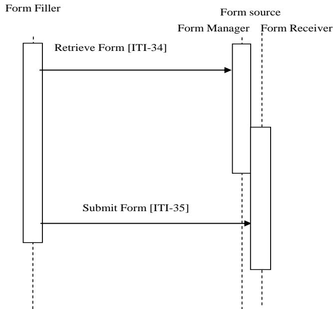
図 17.4-1: Case 1: Retrieve Form と Submit Form ; Form Manager は Form Receiver とグルーピングされている
