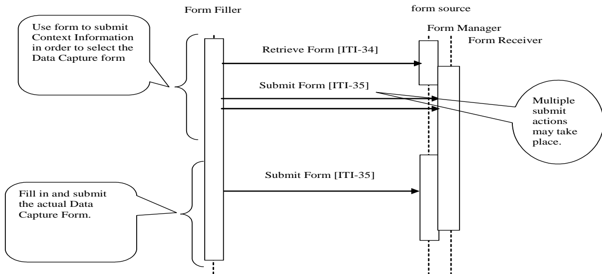
693 図 17.4-4: Case 4: Retrieve Form と Submit Form 694
