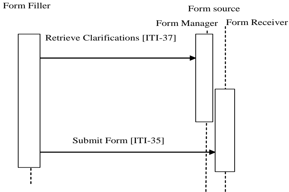
図 17.4-5: Case 5: Clarifications オプションが使用可能な Form Filler
